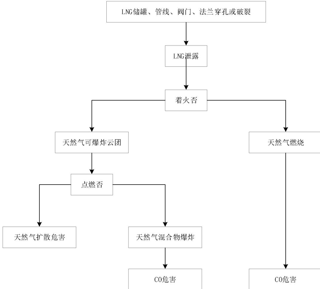
图7-1 LNG液化天然气事故树分析图
