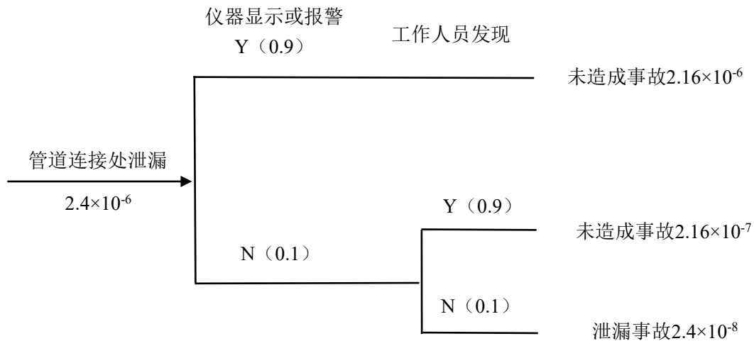
图7-2 项目系统事件树示意图
