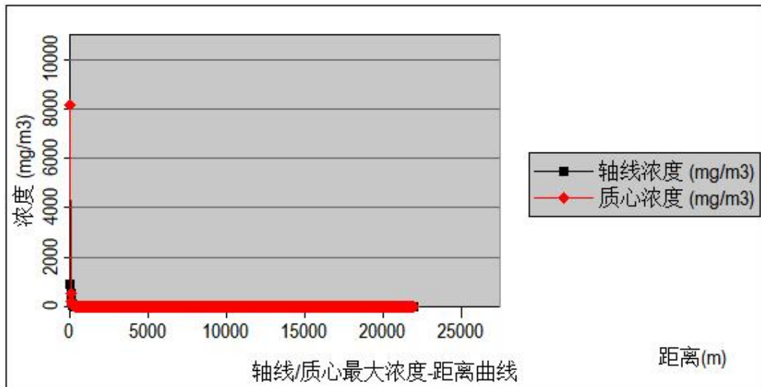
图8-1 LNG管道连接处最大浓度-轴线距离图
