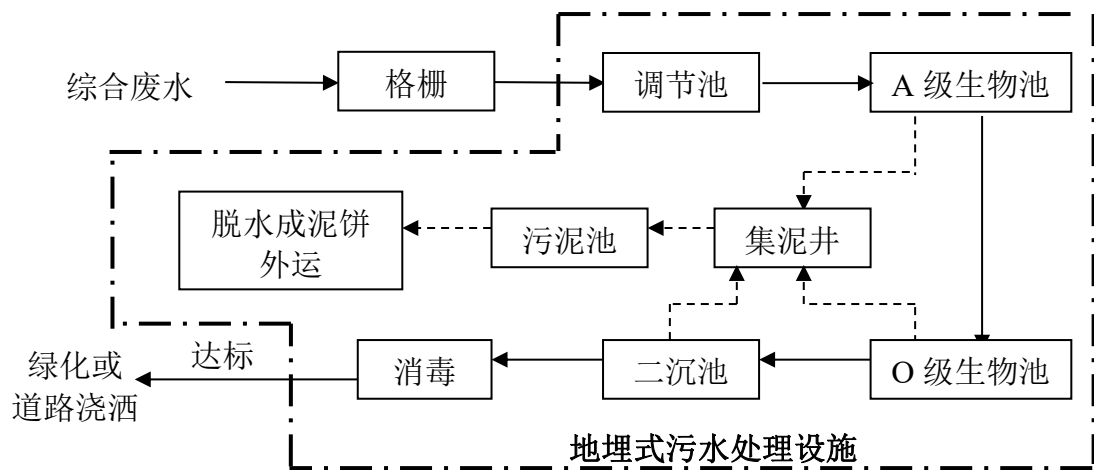
图 4-1 项目污水处理站工艺流程图
