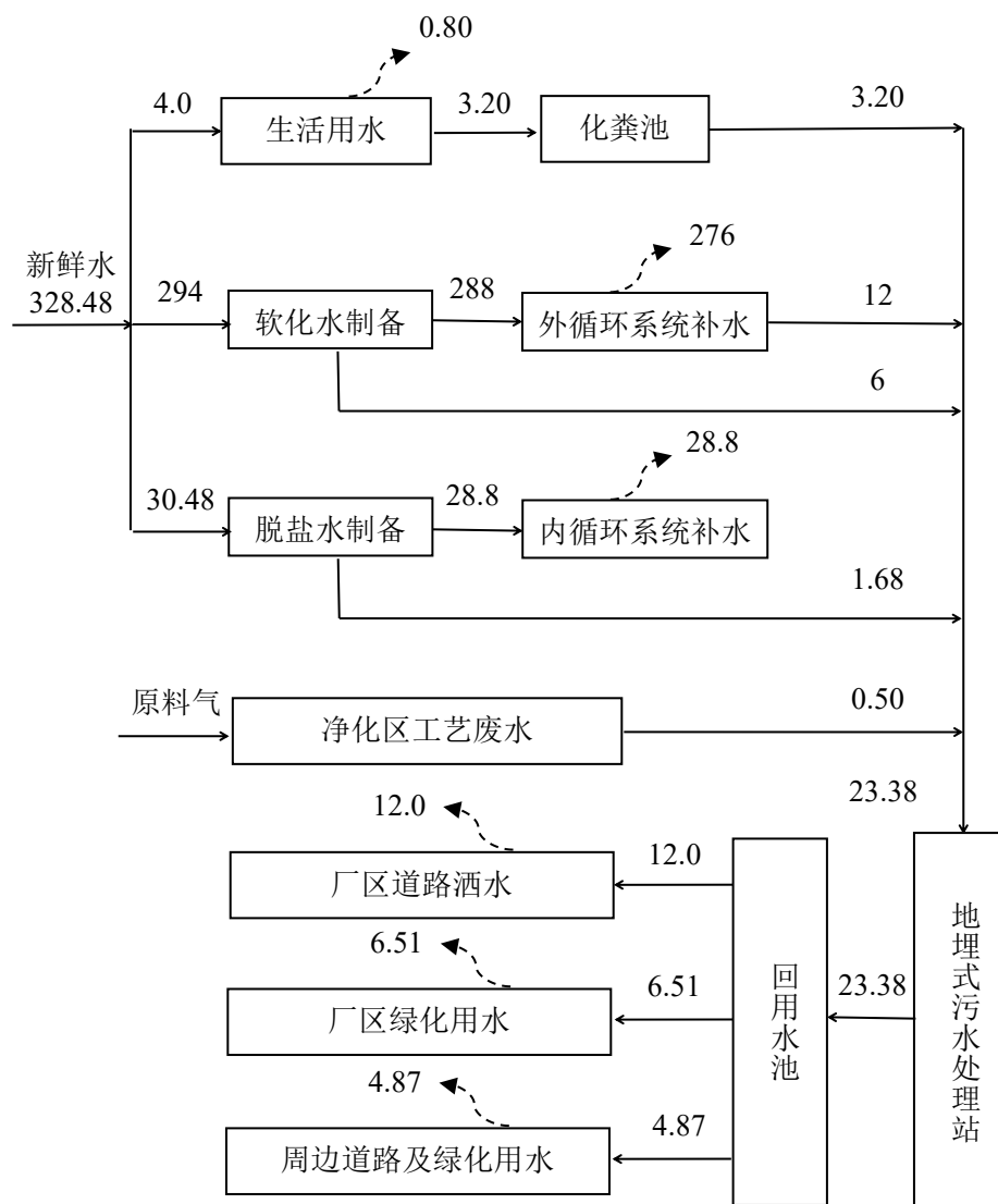
图 2-2 项目非采暖季水平衡图 (m 3 /d)
