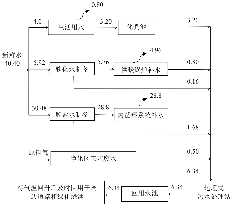
图 2-1 项目采暖季水平衡图 (m 3 /d)
